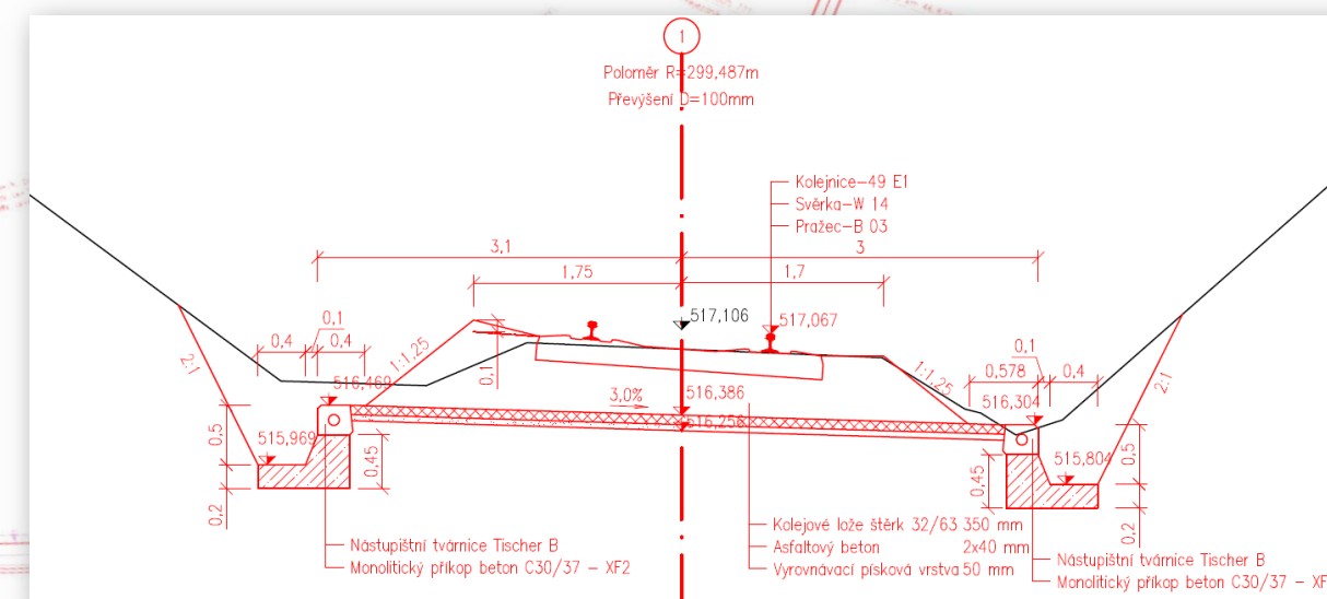
Příčný řez tratí ve skalním zářezu
