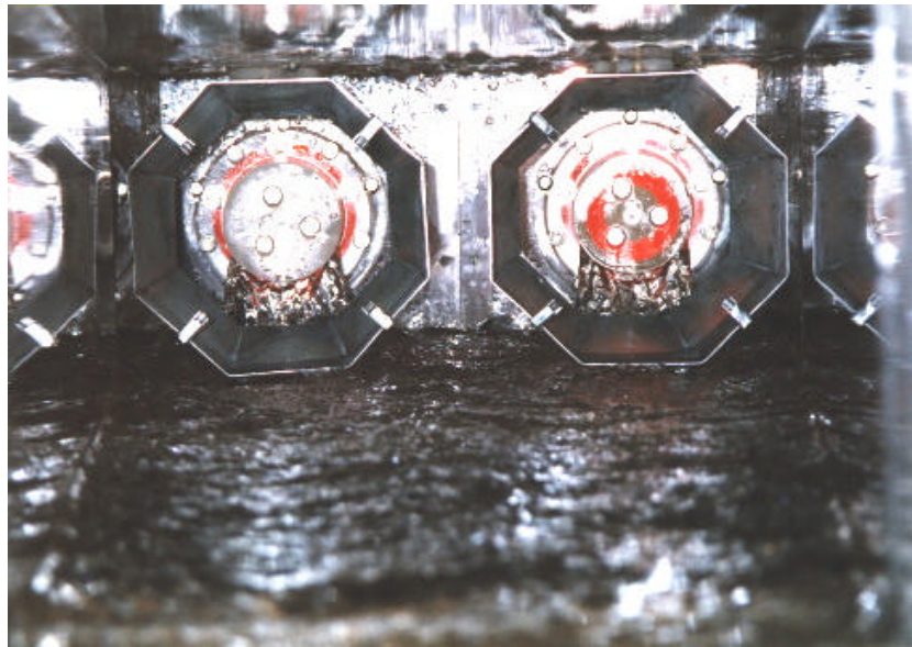
Obr. 6.8 Modely zkoušených usmernovaců výtokových paprsků z rozstrikovacích uzáverů VD Morávka
