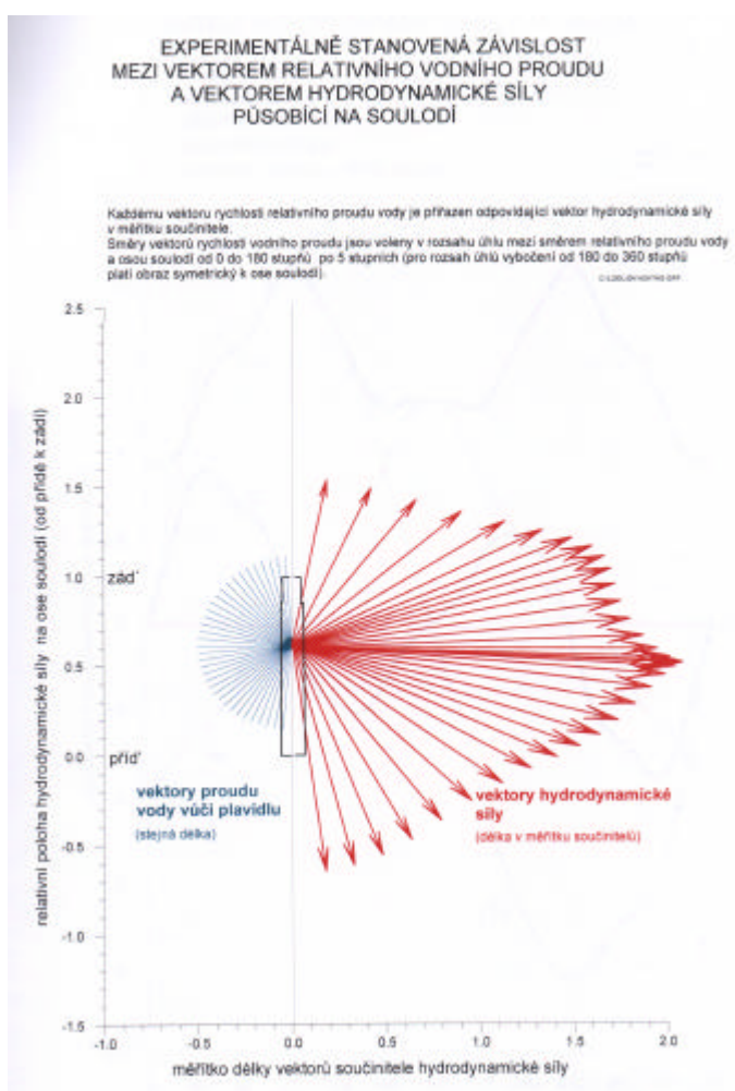
Obr. 6.29 Experimentální stanovení zatížení působícího na plavidlo od hydrodynamického účinku proudu (modelový hydraulický výzkum na žlabu), model soulodí uchycen shora na přesných vahách
