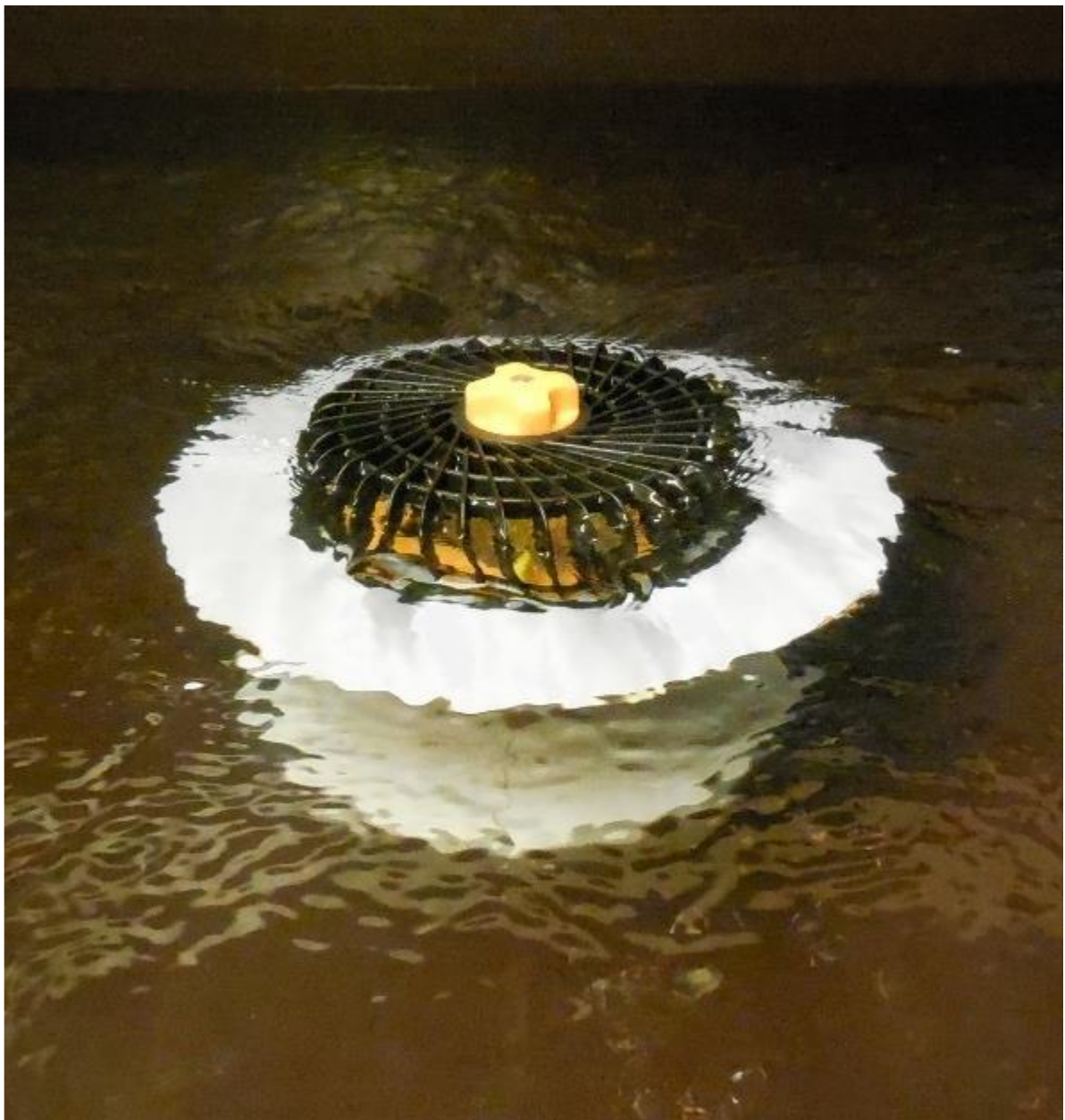
Gravitační vpust s usměřovači proudu
