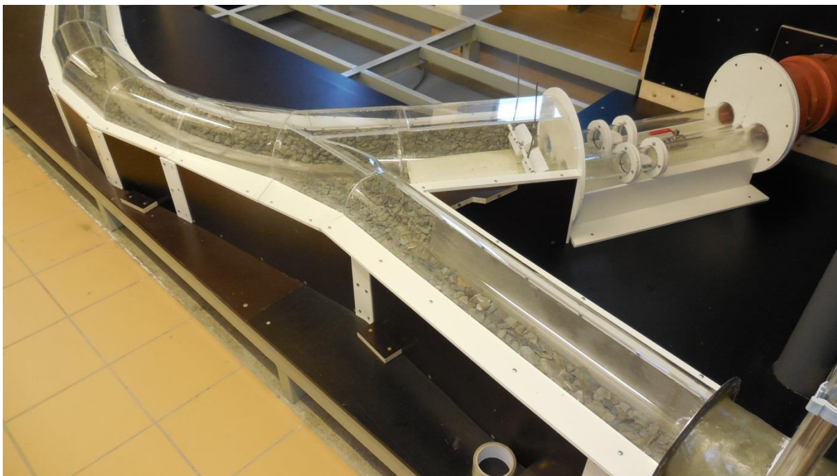
Obtokový tunel
