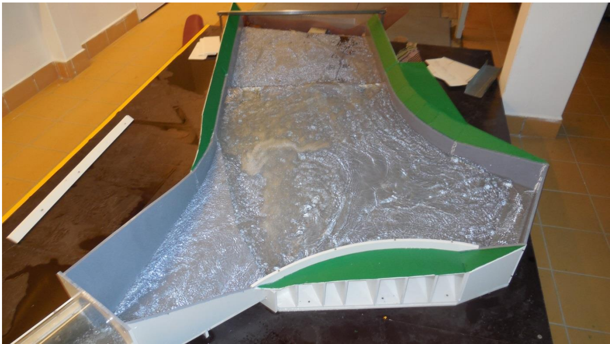
Proudění ve vývaru
