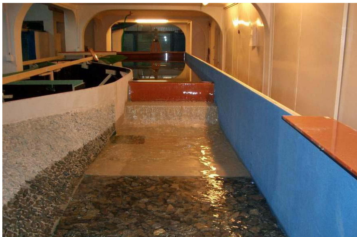
Fyzikální model rybího přechodu
