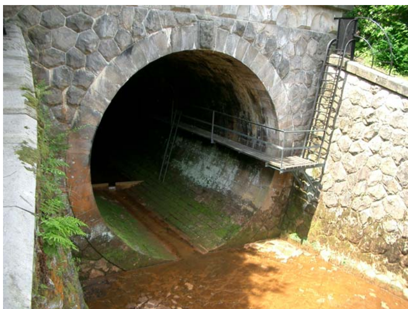
Prostor vyústění pravé obtokové štoly s obdélníkovým přelivem pro měření průsaků
