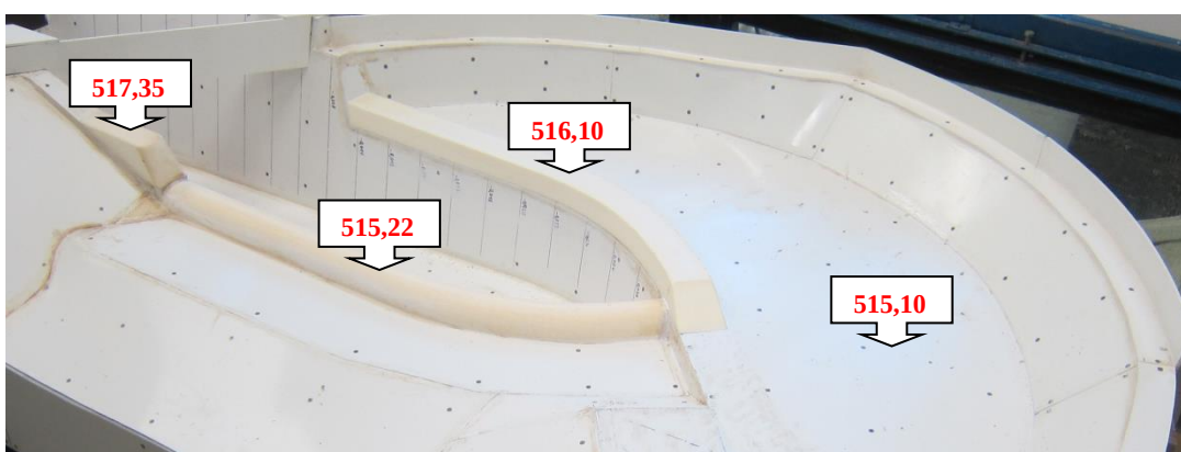
Varianta 2.1. Výškové úrovně po přepočtu na dílo v m n. m
