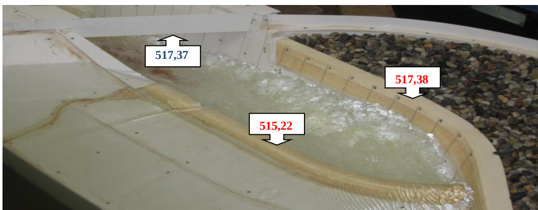
Varianta 1. Výškové úrovně po přepočtu na dílo v m n. m
