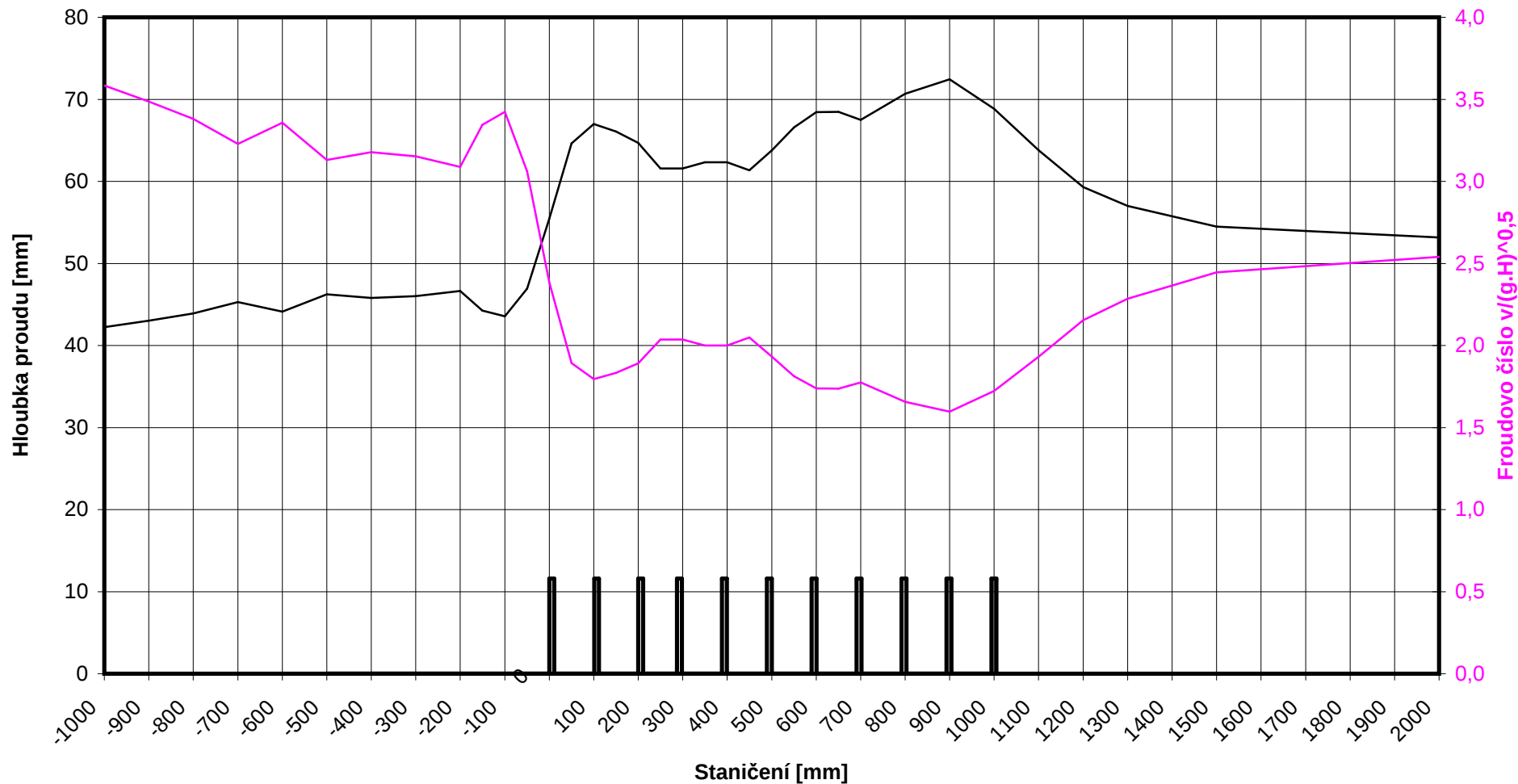
Průběh hloubky proudu - Varianta 6 šířka žlabu 412 mm, sklonu 4,81 %, průtok 40,16 l.s -1 , Re=20930
