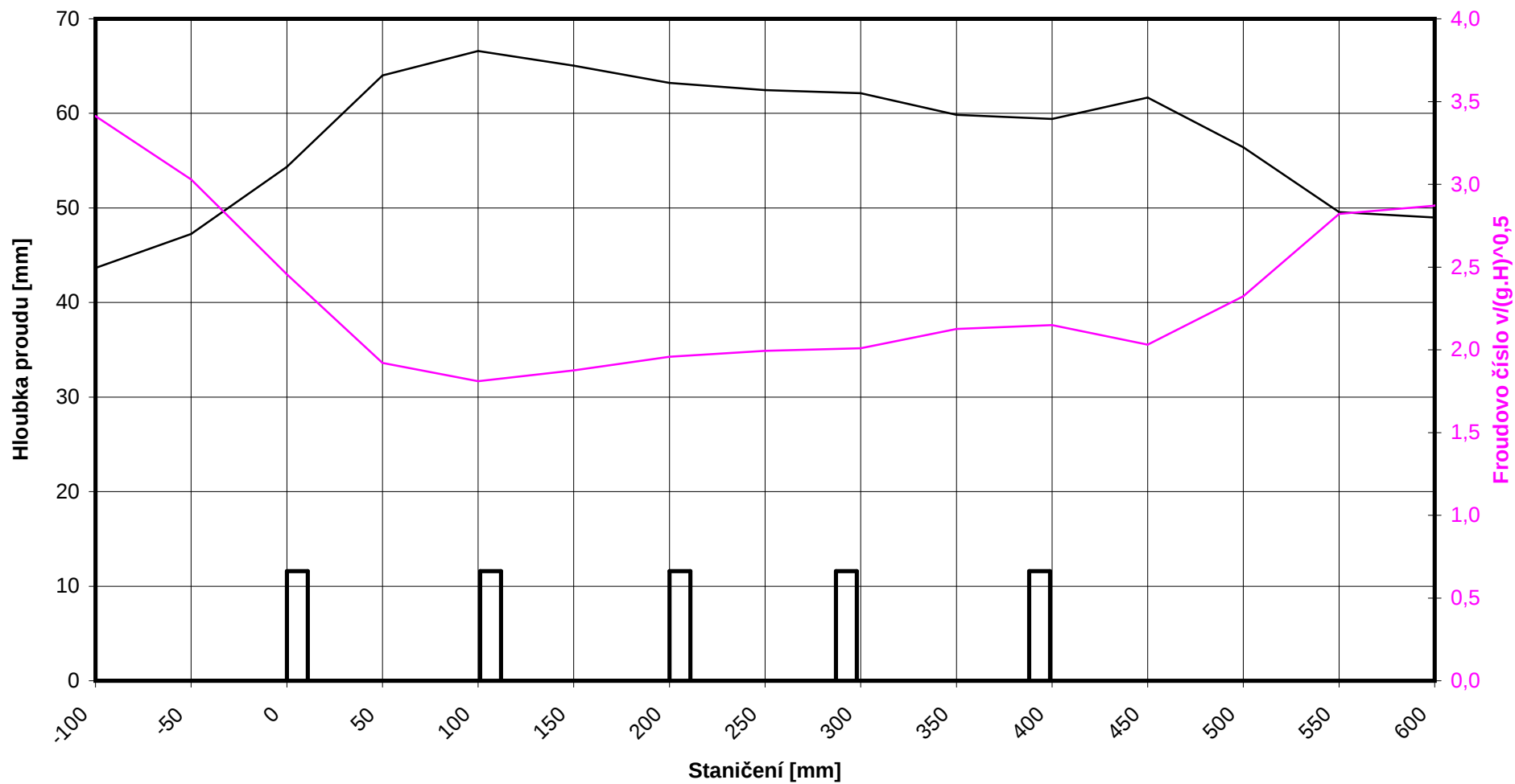
Průběh hloubky proudu - Varianta 4 šířka žlabu 412 mm, sklonu 4,81 %, průtok 40,16 l.s -1 , Re=20930
