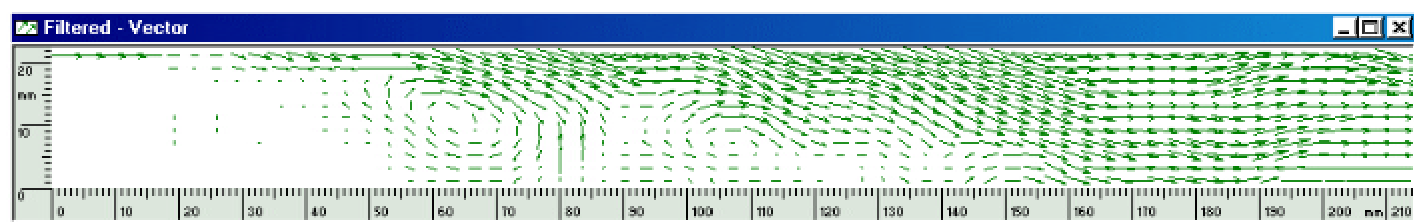
Jeden okamžitý stav rychlostního pole za „schodem“ – náhlým rozšířením průřezného proudu
