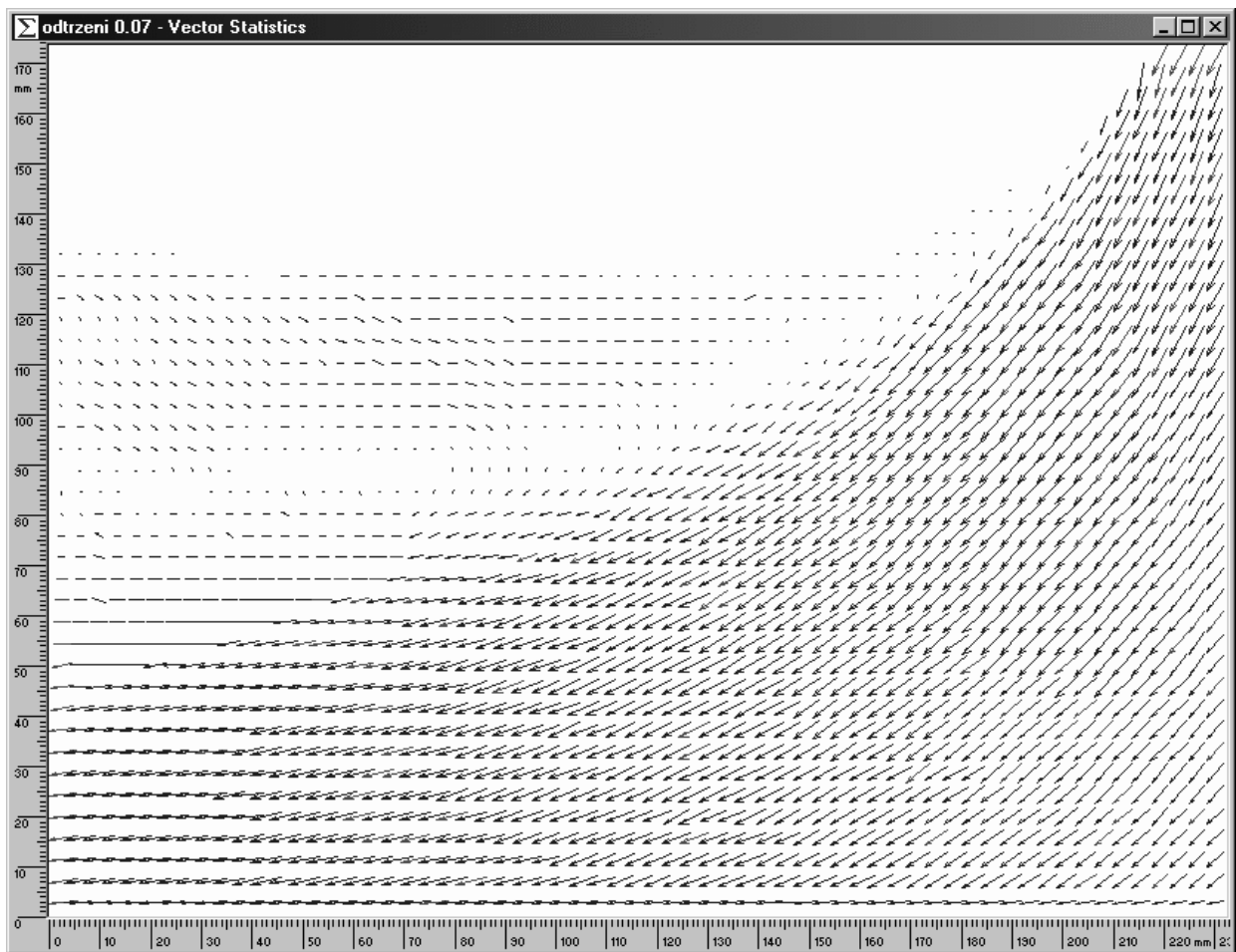
Obr.4 Detail odtržení proudu od stěny
