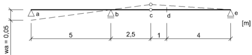
Obr. 6.1: Model konstrukce a zatížení
