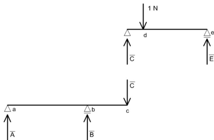
Obr. 6.2: Schéma reakcí vnitřních a vnějších vazeb
