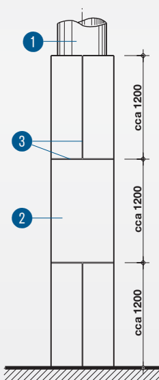
Detail B – uspořádání spár
