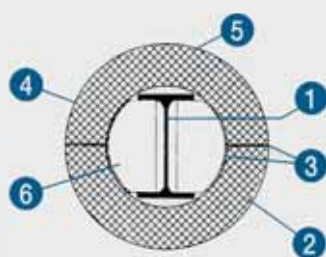
Detail C – provedení na válcovém profilu
