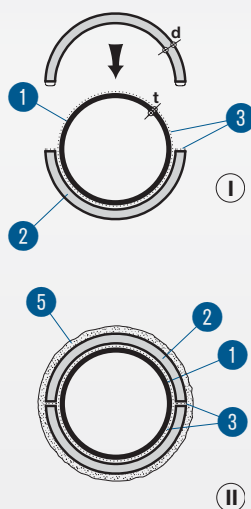
Detail A – průběh montáže
