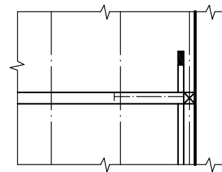
SLOUPEK KOTVEN KE STĚNĚ (PODLOŽENO A 400SH)
