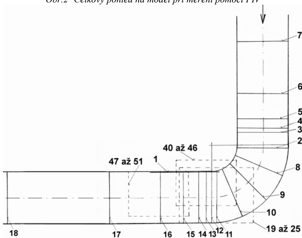
Obr.3 Schéma rozmístění PIV měrných řezů
