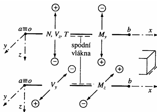
Obr. 4.4: Znaménková konvence pro pořadnice složek vnitřních sil
