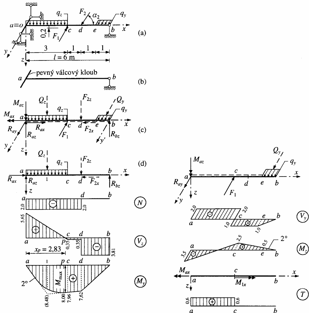
Obr. 4.8: Prostorově namáhaný vodorovný nosník
