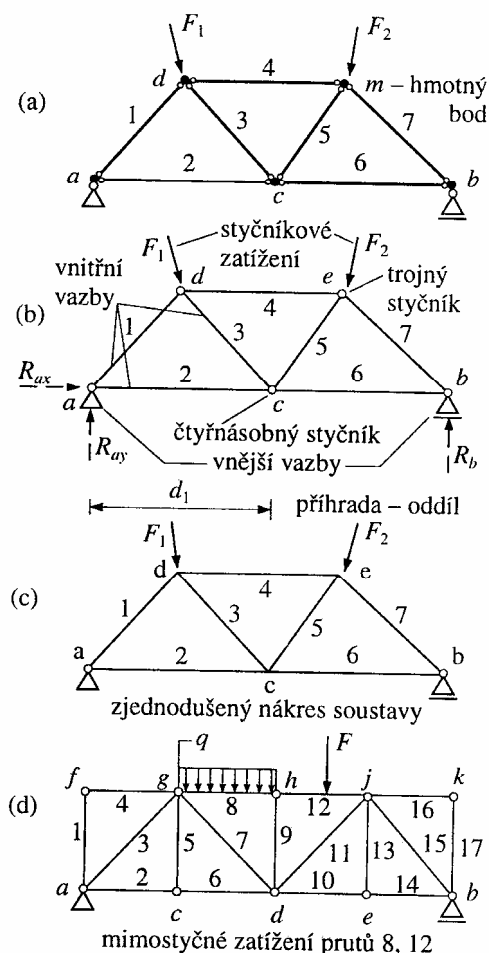
Obr. 3.1: Rovinná kloubová prutová soustava
