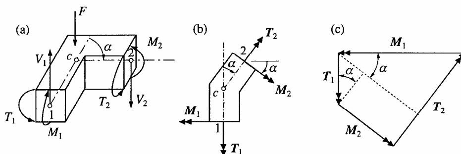
Obr. 4.6: Uvolněný uzel balkonového nosníku
