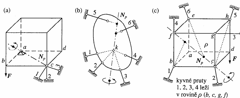
Obr. 4.1: Výjimečné případy podepření tuhého tělesa
