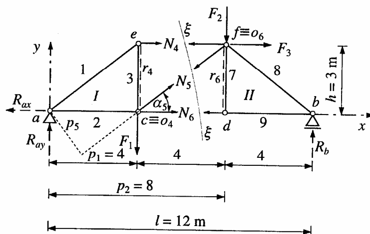
Obr. 3.9: Rozdělení prutové soustavy na dvě části
