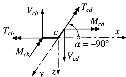
Obr. 4.12: Uvolněný uzel c balkonového nosníku
