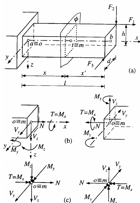
Obr. 4.2: Složky výslednice vnitřních sil
