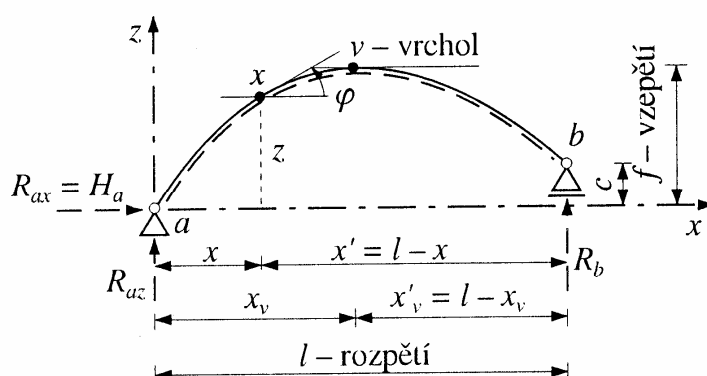
Obr. 2.1: Rovinný zakřivený nosník
