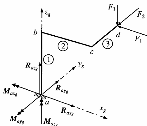
Obr. 4.9: Prostorově lomený konzolový nosník
