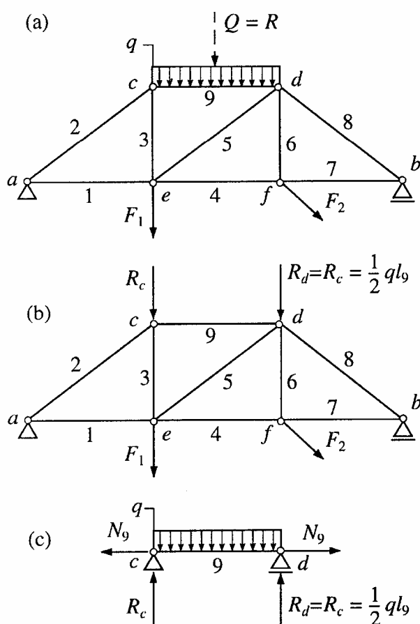
Obr. 3.14: Mimostyčné zatížení prutové soustavy
