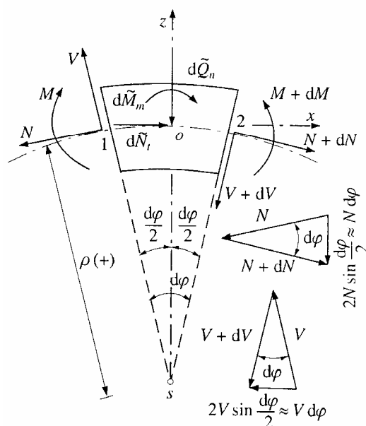
Obr. 2.4: Zakřivený prutový element
