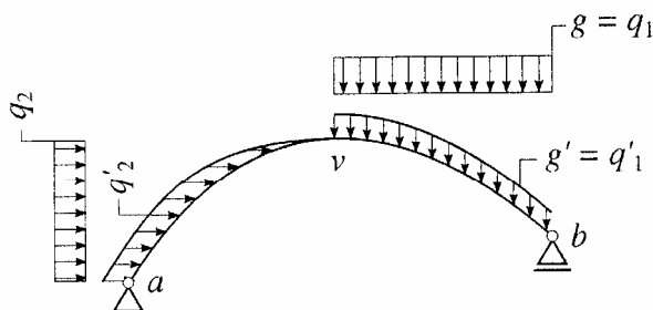
Obr. 2.2: Spojitá zatížení na zakřiveném nosníku
