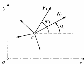
Obr. 3.7: Obecný styčník se zatížením
