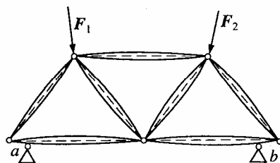
Obr. 3.2: Příhradový nosník
