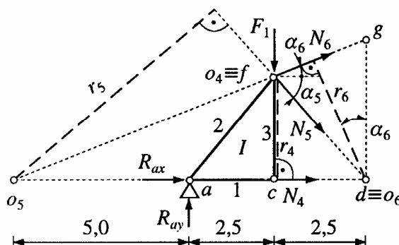
Obr. 3.10: Uvolněná část prutové soustavy
