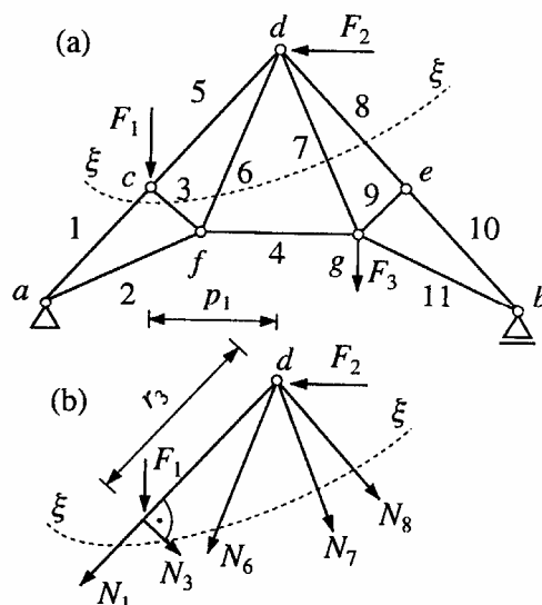
Obr. 3.12: Zvláštní případ průsečné metody
