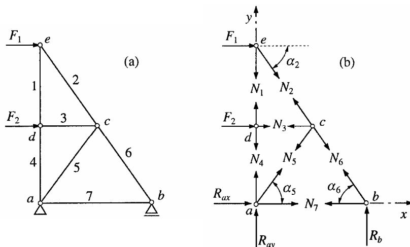
Obr. 3.6: Uvolněné styčnický prutové soustavy
