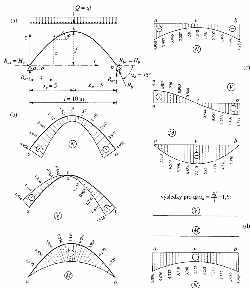
Obr. 2.5: Prostý nosník s parabolickou střednicí
