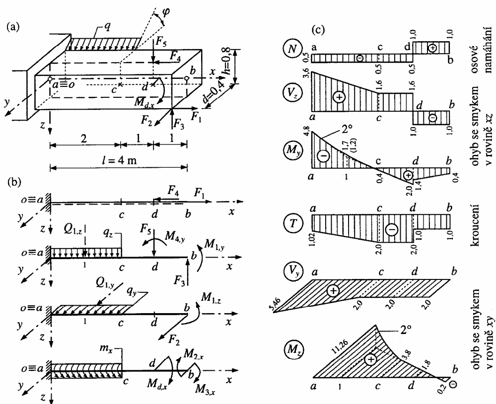
Obr. 4.7: Vodorovný konzolový nosník prostorově zatížený
