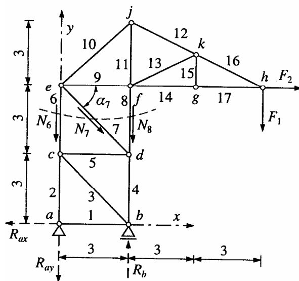
Obr. 3.11: Prutová soustava k příkladu 3.3
