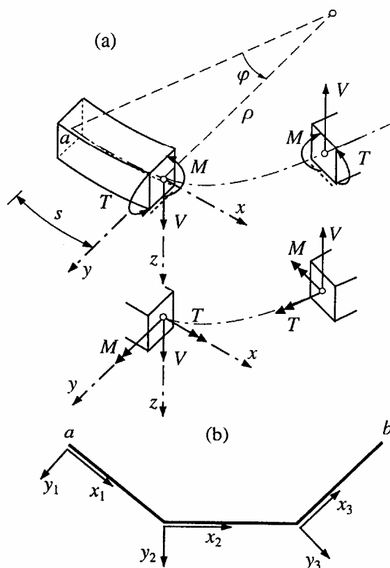
Obr. 4.5: Zakřivený a lomený balkonový nosník
