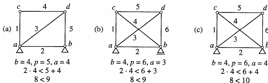
Obr. 3.3: Staticky neurčité kloubové prutové soustavy
