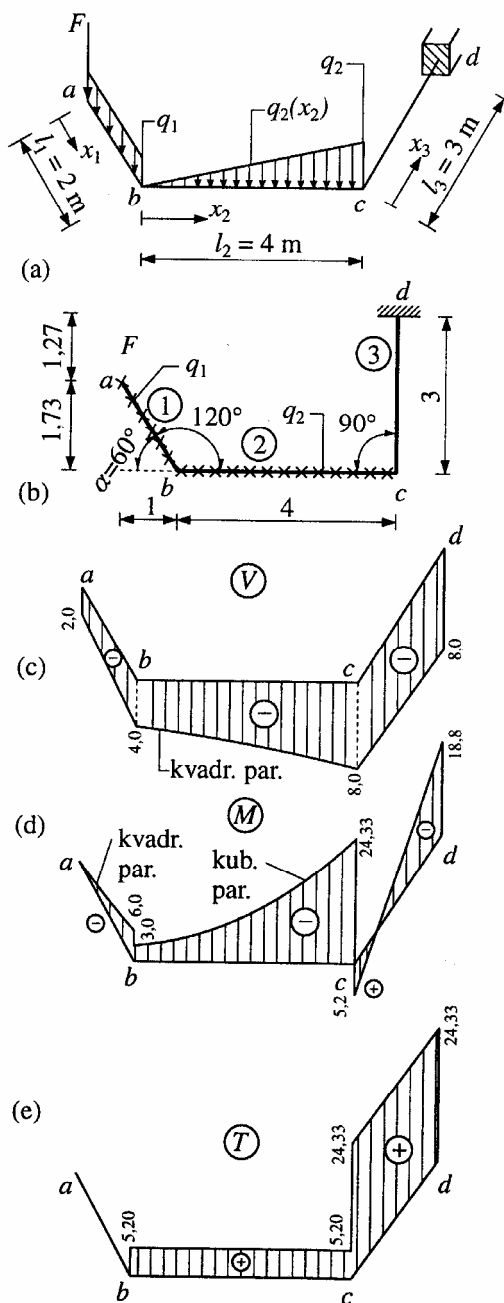
Obr. 4.11: Konzolový lomený balkonový nosník
