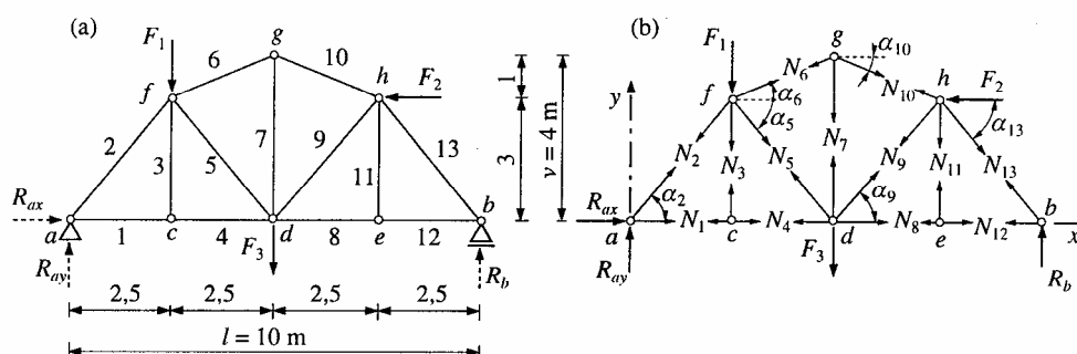
Obr. 3.8: Prutová soustava řešená zjednodušenou styčnickovou metodou
