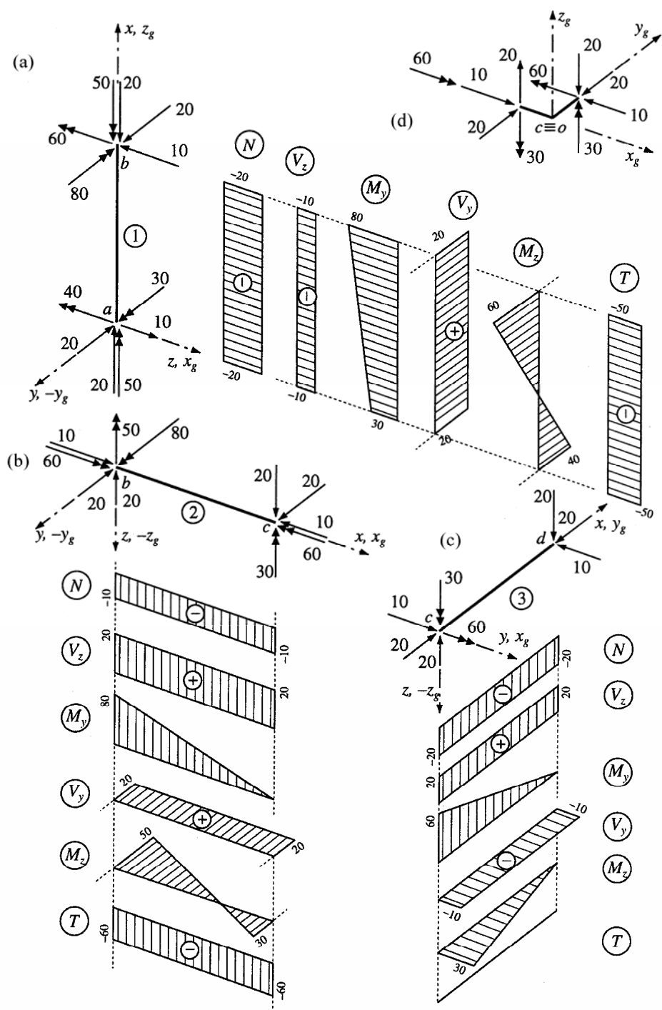
Obr. 4.10: Průběhy složek vnitřních sil na jednotlivých prutech nosníku v lokálních souřadnicových soustavách
