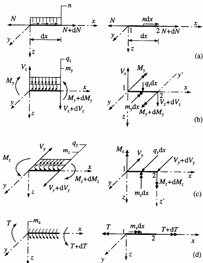
Obr. 4.3: Nosníkový element s vnějším zatížením a složkami vnitřních sil
