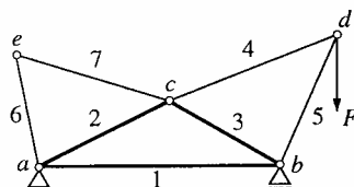
Obr. 3.5: Trojúhelníková prutová soustava
