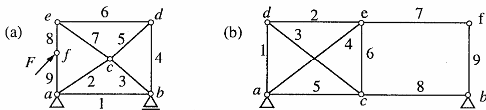
Obr. 3.4: Výjimečné případy kloubových prutových soustav
