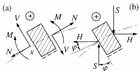
Obr. 2.3: Složky vnitřních sil zakřiveného prutu
