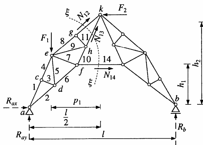
Obr. 3.13: Kombinace styčnickové a průsečné metody
