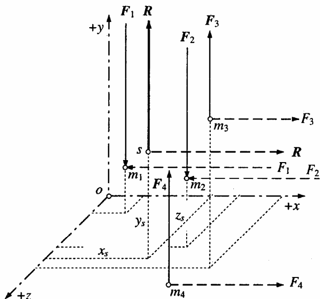
Obr. 4.12: Statický střed soustavy rovnoběžných sil v prostoru
