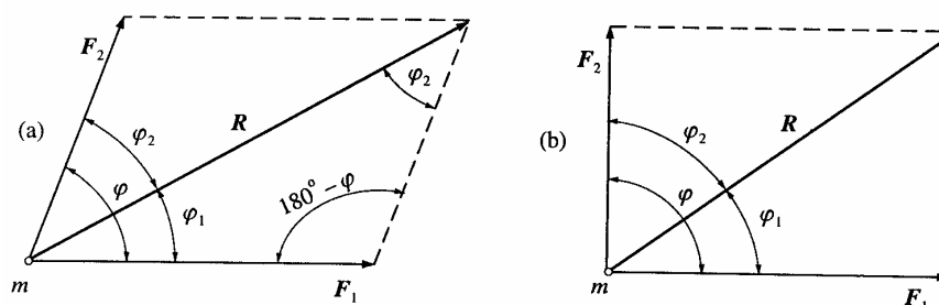
Obr. 3.2: Dvě síly se společným působištem
