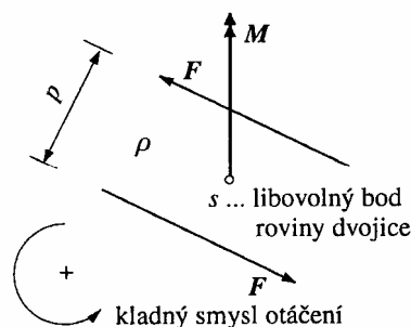
Obr. 2.6: Dvojice sil
