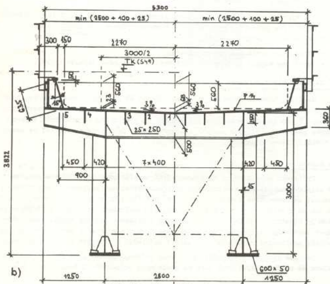
Obr. 9.1 Dispoziční výkres
