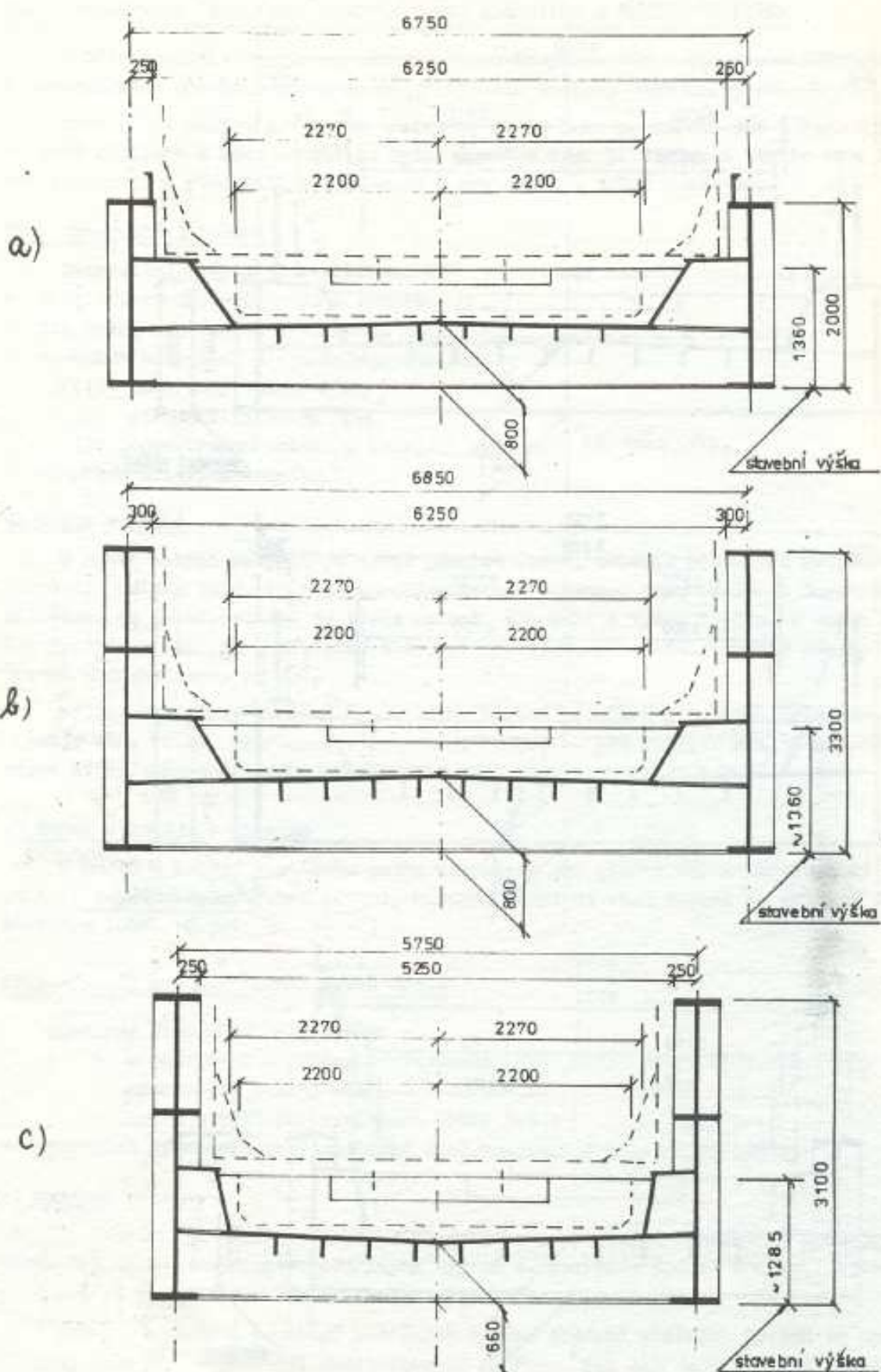
Obr. 10.2 Dispoziční řešení mostů rozpětí cca 25,0 až 35,0 m
