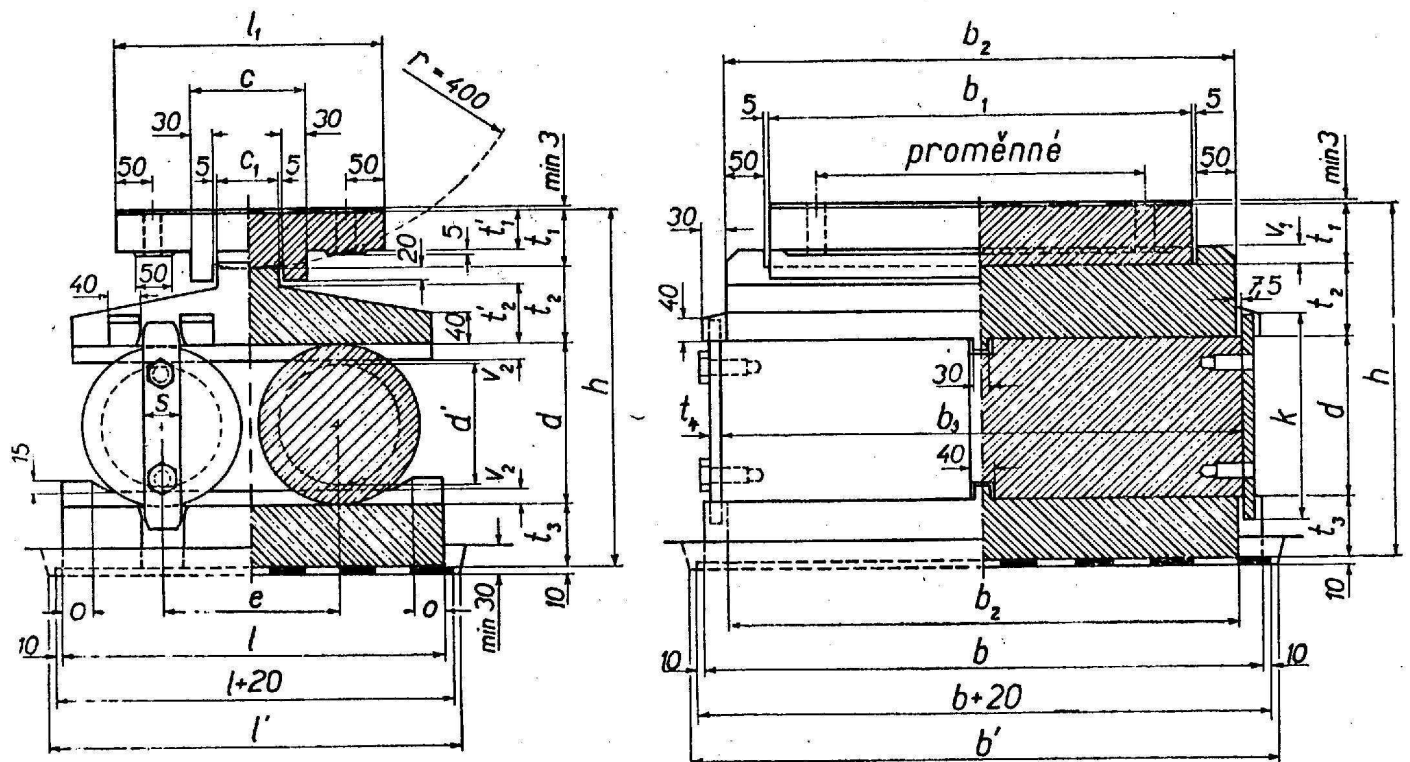
Obr. 8. Dvouřádkové ložisko
