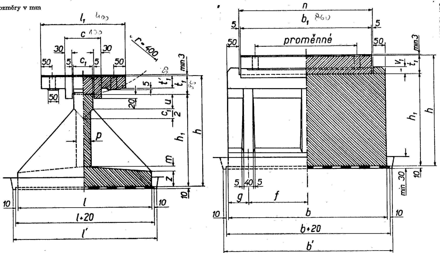
Obr. 7. Pevné ložisko
